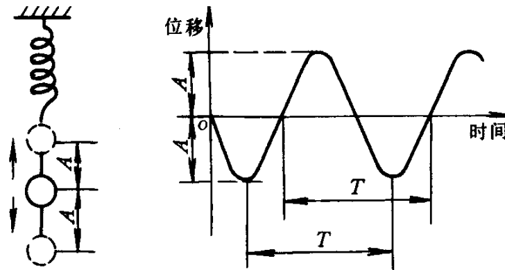
图 1-1 加载弹簧的振动
